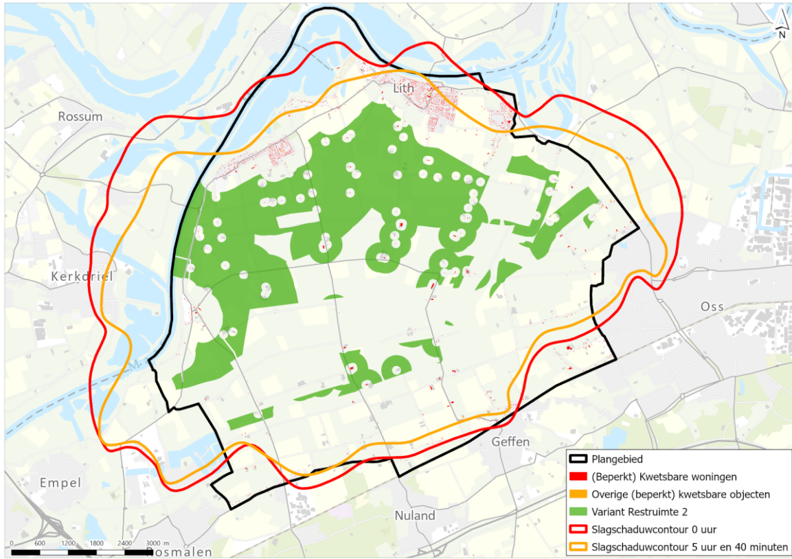
Afbeelding 8.2 Slagschaduwcontouren variant Restruiimte 2
